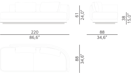
FWATC.RA02 {versão direita} Terminal de Conexão 2,5 Lugares
