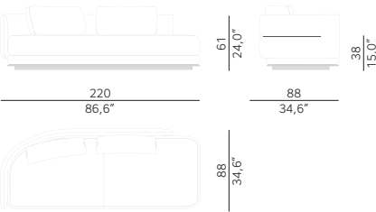
FWATC.LA02 {versão esquerda} Terminal de Conexão 2,5 Lugares
