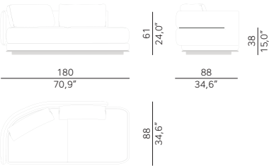
FWATC.LA01 {versão esquerda} Terminal de Conexão 2 Lugares
