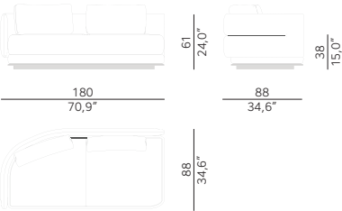
FWATU.LA01 {versão esquerda} Terminal de União 2 Lugares
