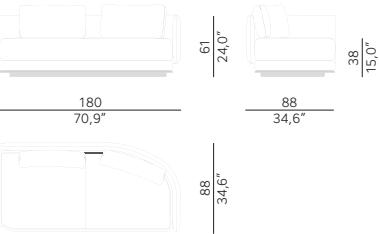
FWATU.RA01 {versão direita} Terminal de União 2 Lugares
